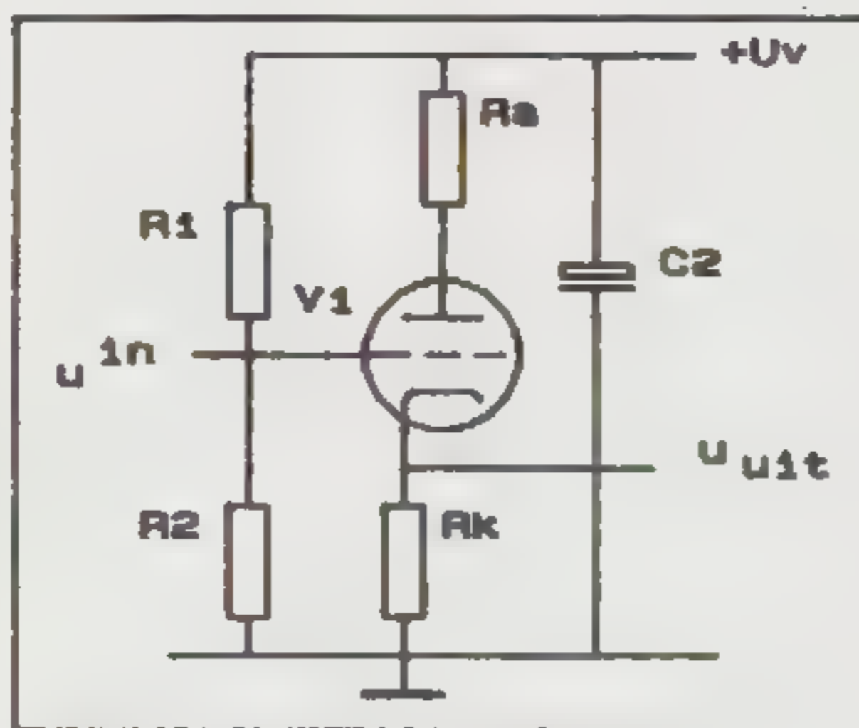
Figuur 19 Kathodevolger
